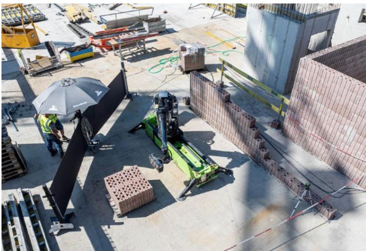
Der Roboter mauert auf der Baustelle des Projekts Kladno Living in Tschechien © PORR/Jan Hrdý
